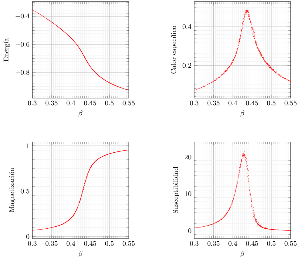
Figure 2: Resultados obtenidos del archivo simulations_L032.txt
