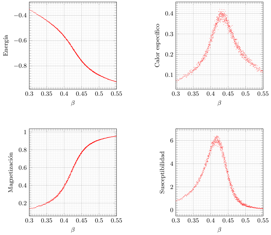
Figure 1: Resultados obtenidos del archivo simulations_L016.txt
