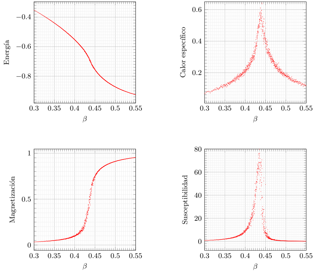
Figure 3: Resultados obtenidos del archivo simulations_L064.txt
