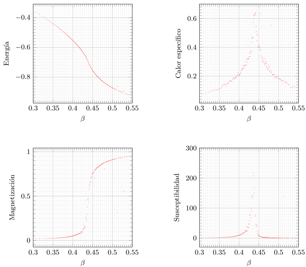
Figure 4: Resultados obtenidos del archivo simulations_L128.txt
